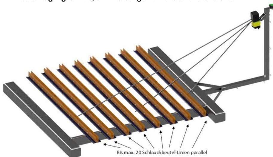
Abb.: Ansicht AIT Pack, Track & Check Bildverarbeitungslösung Schlauchbeutelverpackungsanlagen
