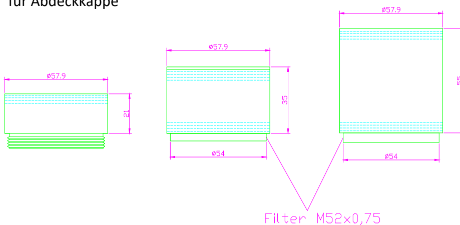
Verlängerung für Abdeckkappe
