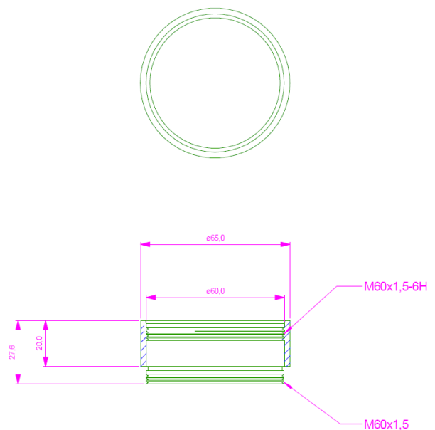
AIT Verlängerung für Abdeckkappe 65mm
