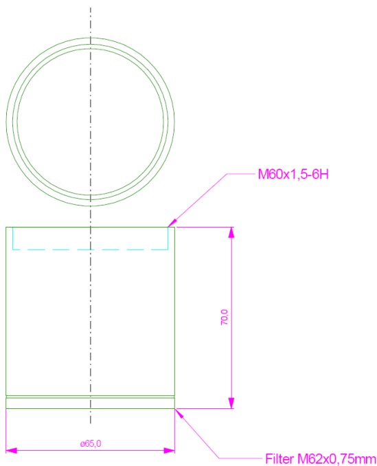
Abdeckkappe 65mm
